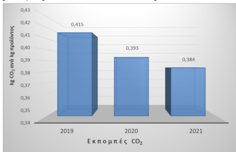
Διάγραμμα 16: Εκπομπές Διοξειδίου του Άνθρακα (CO 2 )
