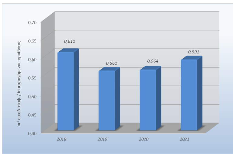
Διάγραμμα 13: Δείκτης Βιοποικιλότητας
