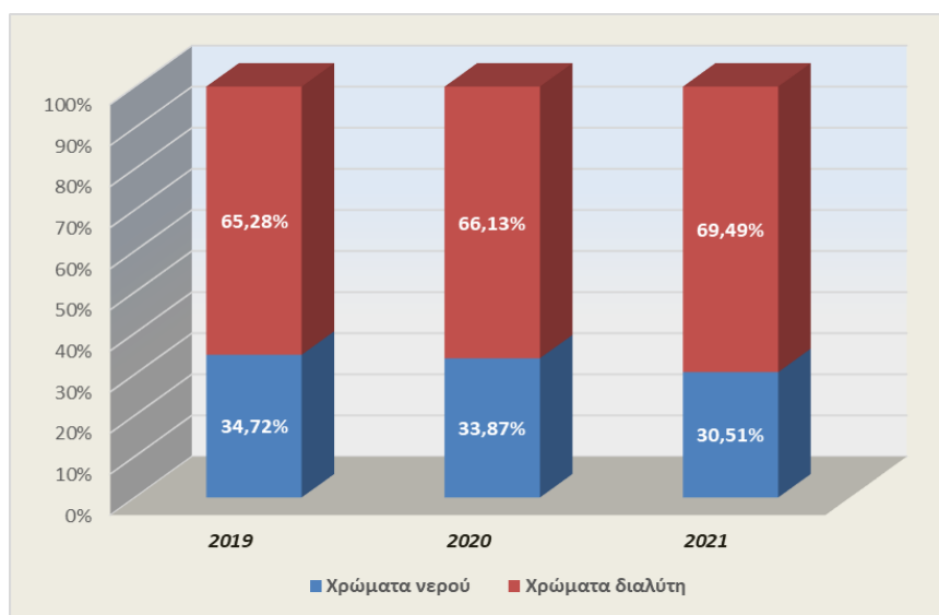
Διάγραμμα 7: Ποσοστό χρήσης χρωμάτων νερού 2019-2020-2021
