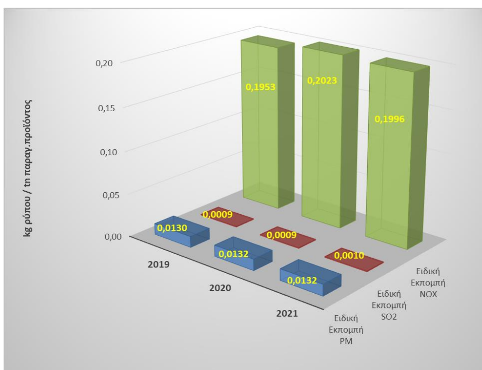
Διάγραμμα 17: Ειδικές Εκπομπές NO x , SO 2 και PM
