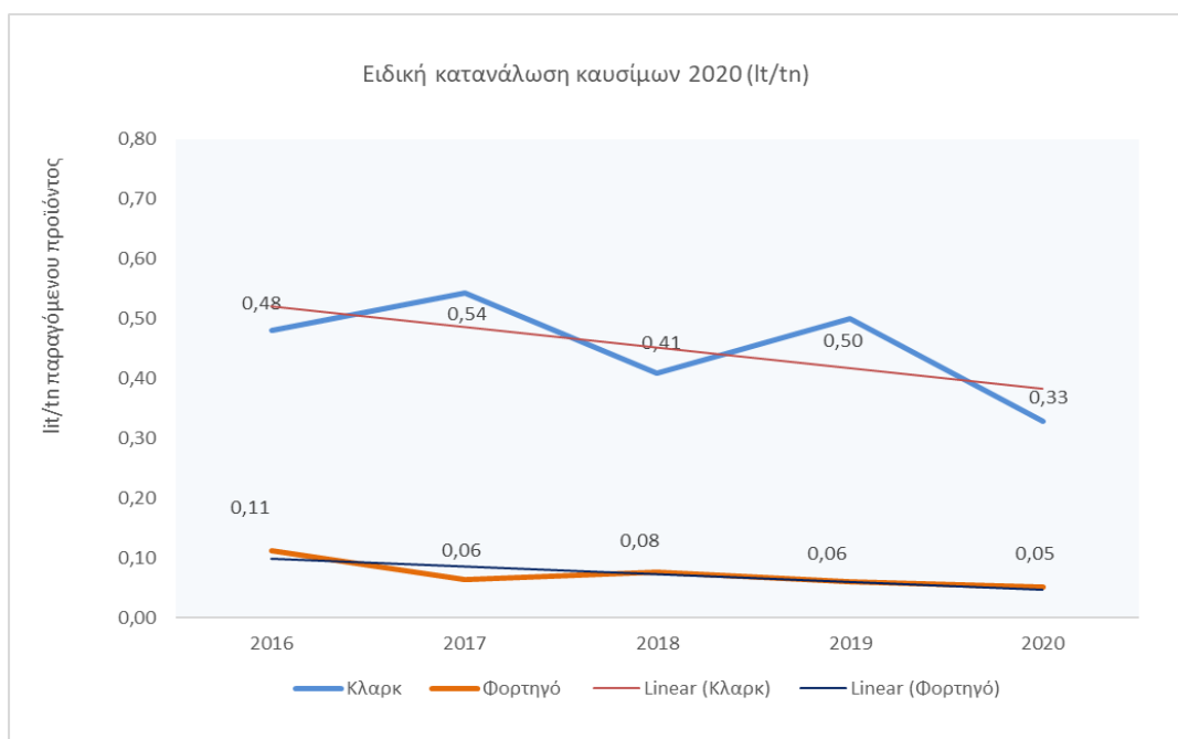
Διάγραμμα 15: Ειδική κατανάλωση καυσίμων
